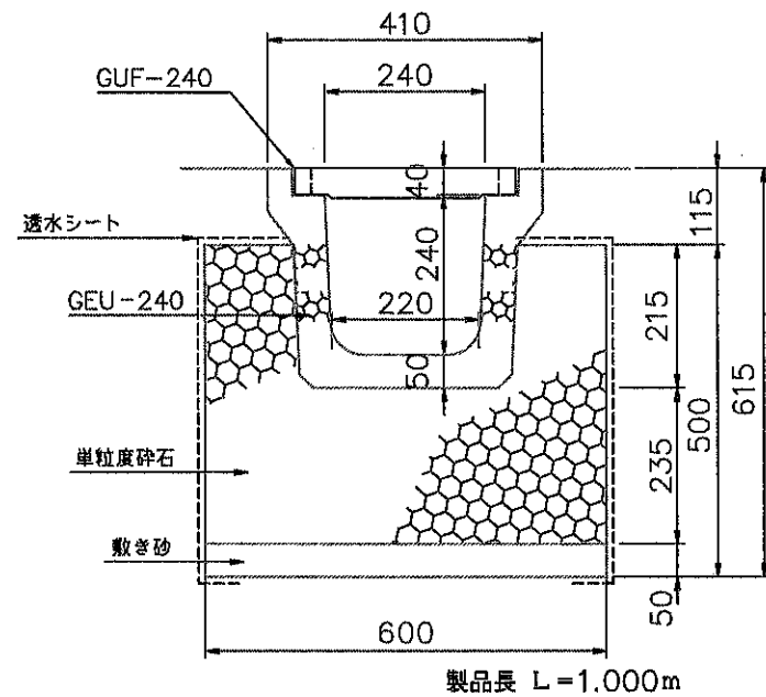
浸透側溝GEU-240構造図 S=1/10
