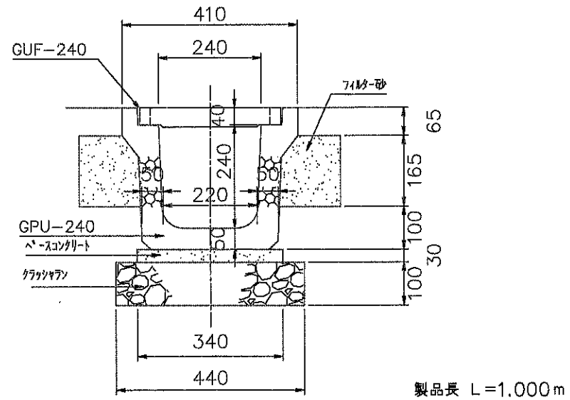
透水側溝GPU-240構造図 S=1/10
