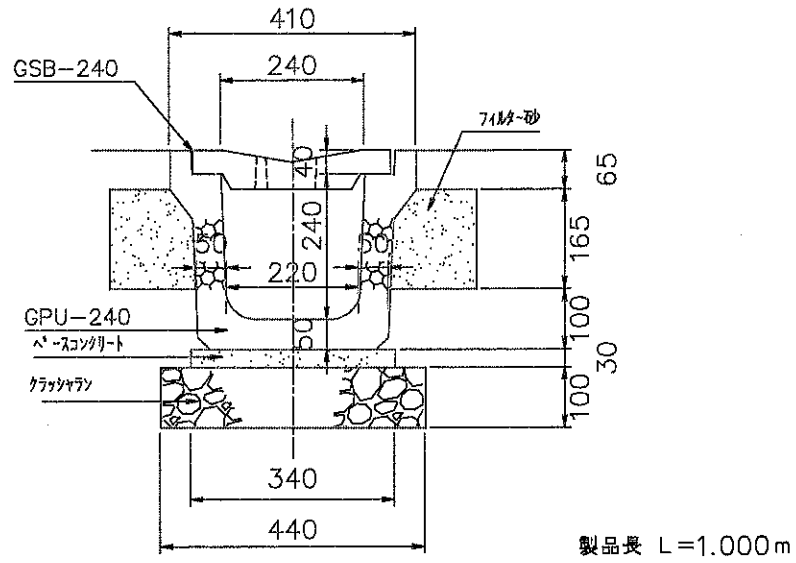
透水側溝GPU-240構造図 S=1/10
